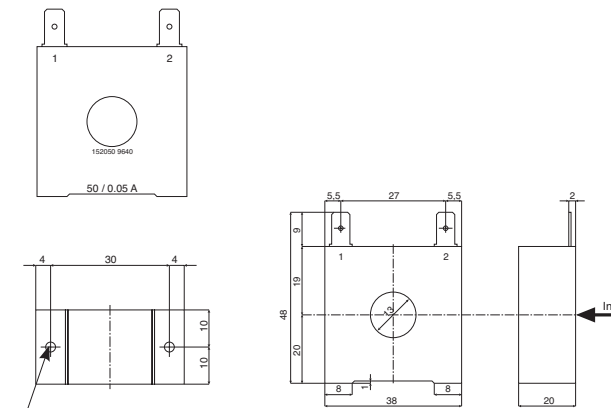
Befestigungsbohrung für Blechschrauben: 2,9 x 9
